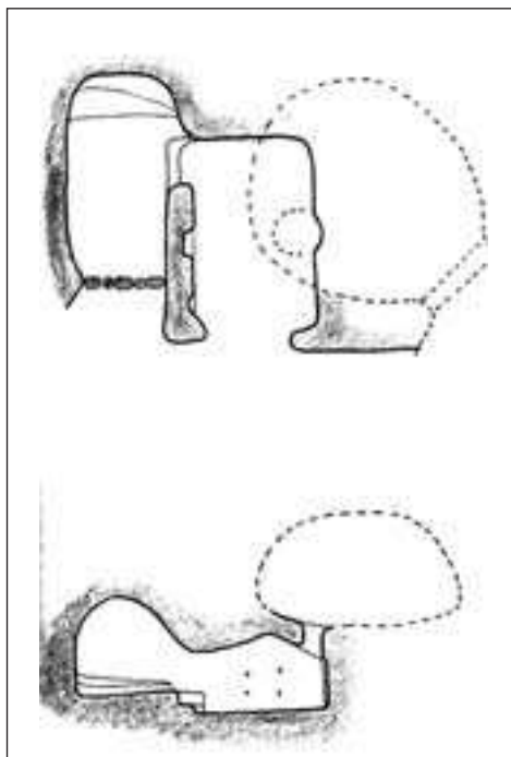
Fig. 14 - Caccuri, planimetria e sezione di un'unità rupestre.
