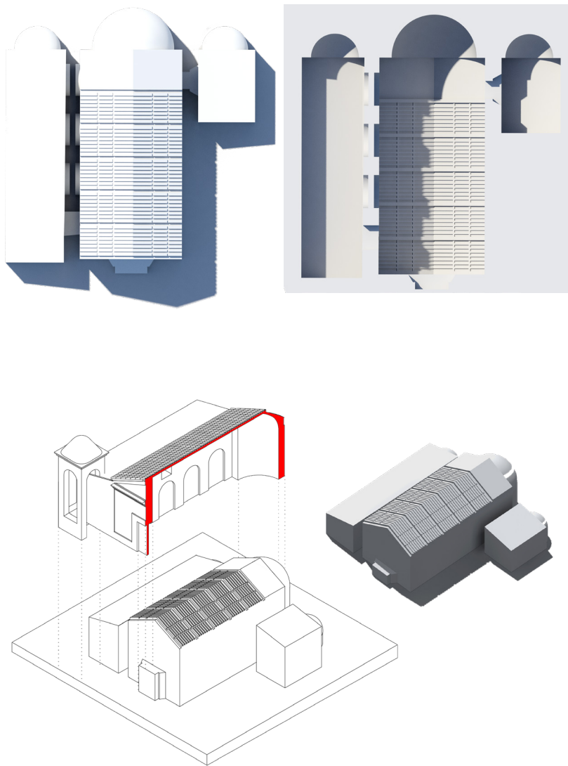
Rappresentazione tridimensionale vuoti/pieni del manufatto
