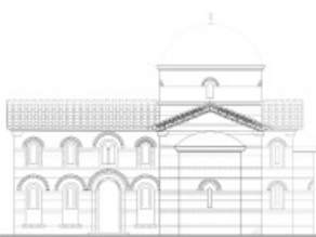
prospetto est
