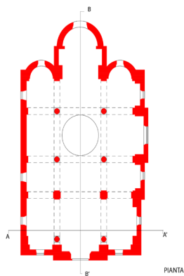
PIANTA
