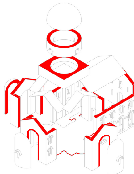
Esploso assonometrico
