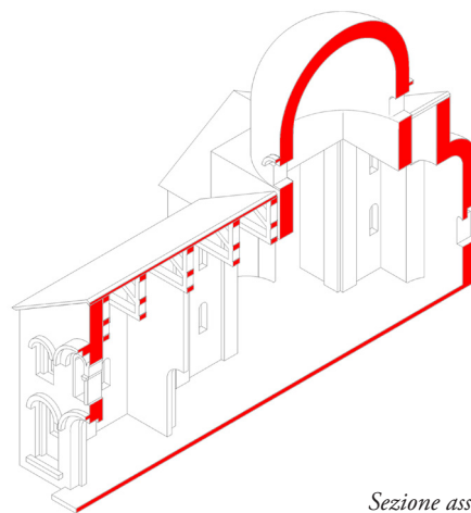
Sezione assonometrica
