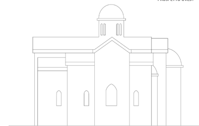
PROSPETTO EST
