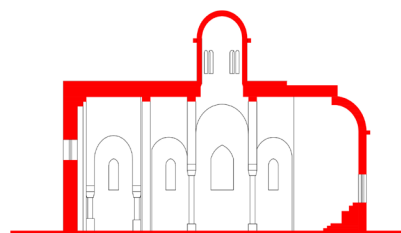
PROSPETTO OVEST
