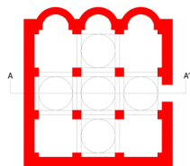
pianta ipotesi 1
