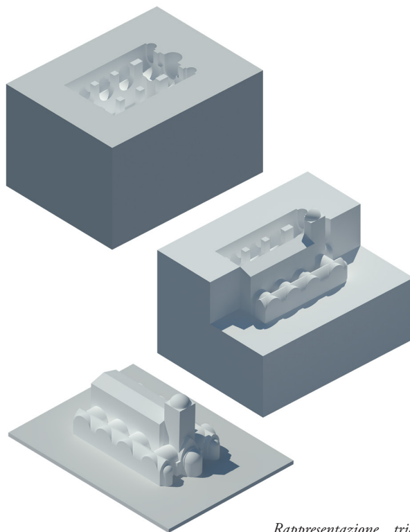
Rappresentazione tridimensionale vuoti/pieni del manufatto
