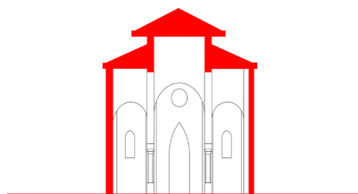
SEZIONE A-A'
