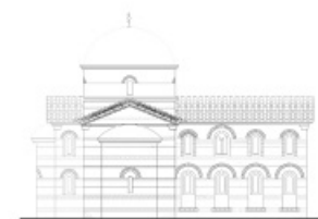
prospetto ovest
